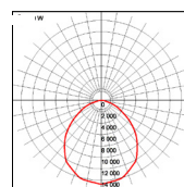
200W-5000K-50x90°
